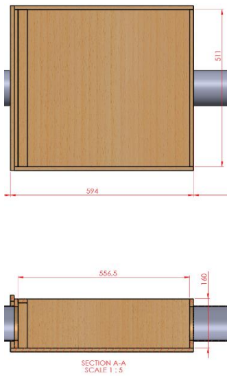
Obrázok 3 Rozmery meracieho boxu
