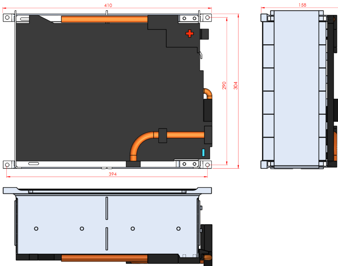
Obrázok 4 Rozmery Batériového modulu BMW i3
