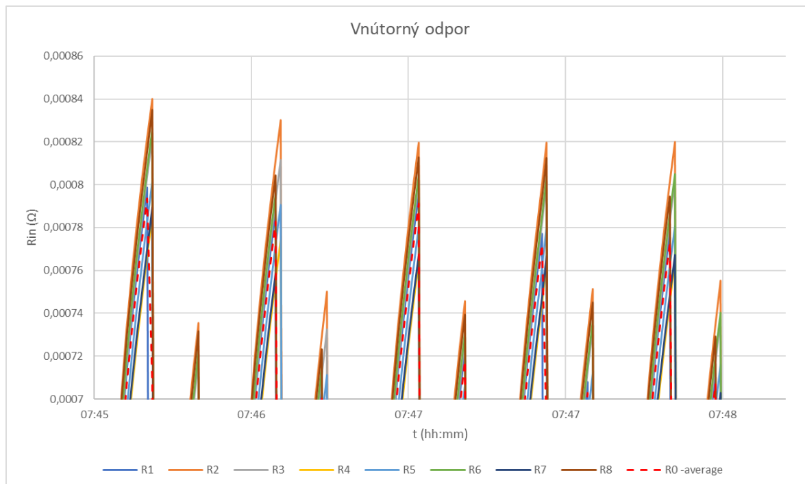
Obrázok 7 Graf určenia vnútorného odporu článkov
