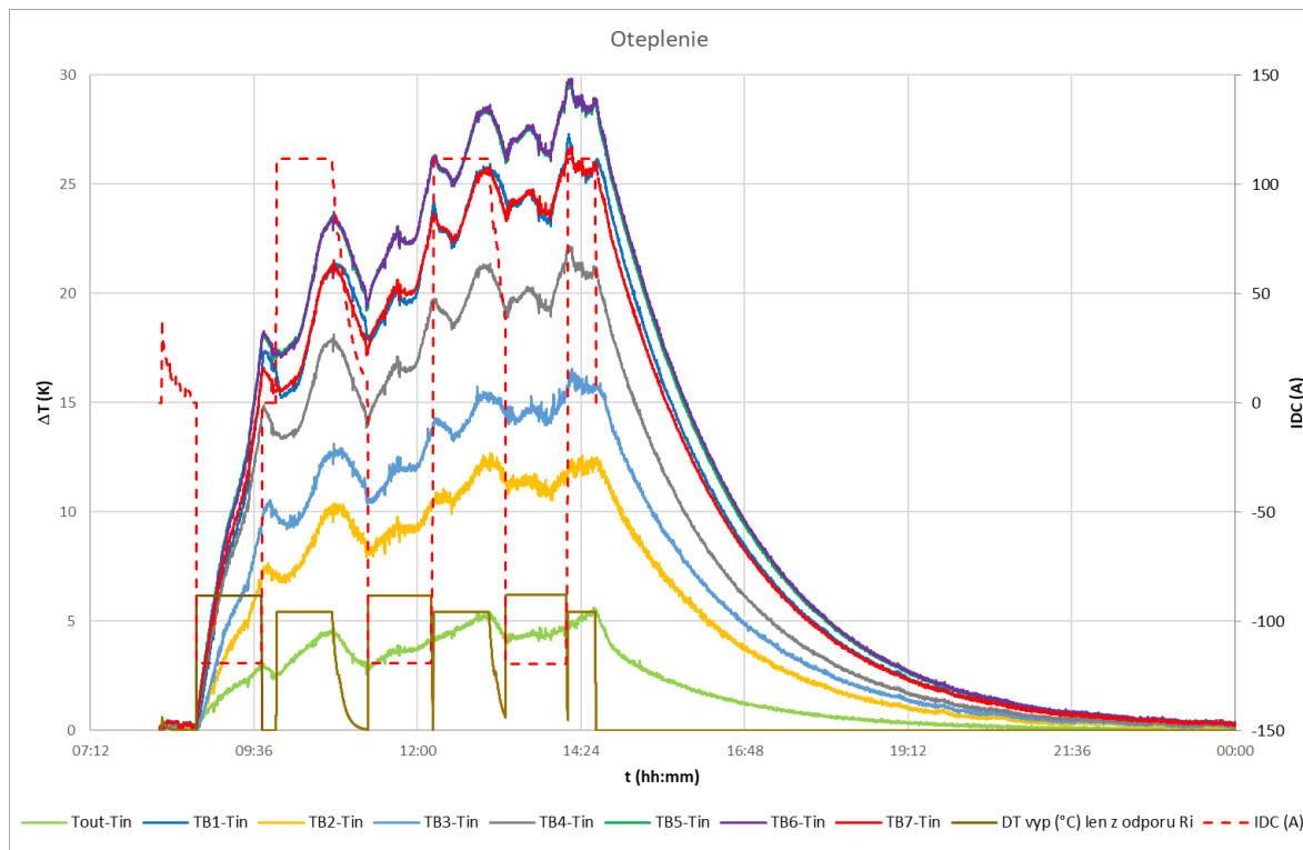
Obrázok 6 Časový priebeh oteplenia článkov a výstupného vzduchu počas cyklického nabíjania a vybíjania modulu prúdom I_{DC}
