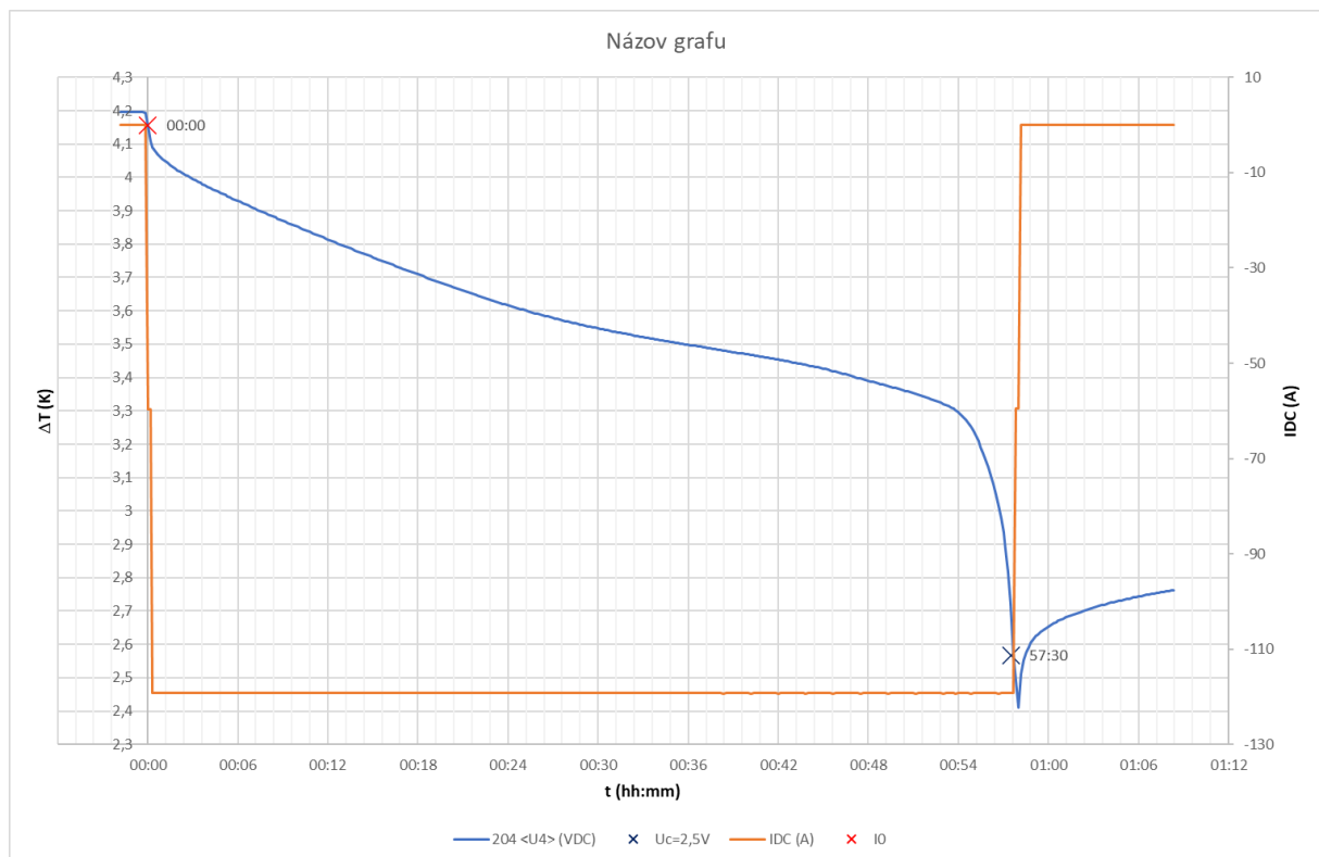
Obrázok 5 Časový priebeh napätia a prúdu článku U3 počas vybíjania
