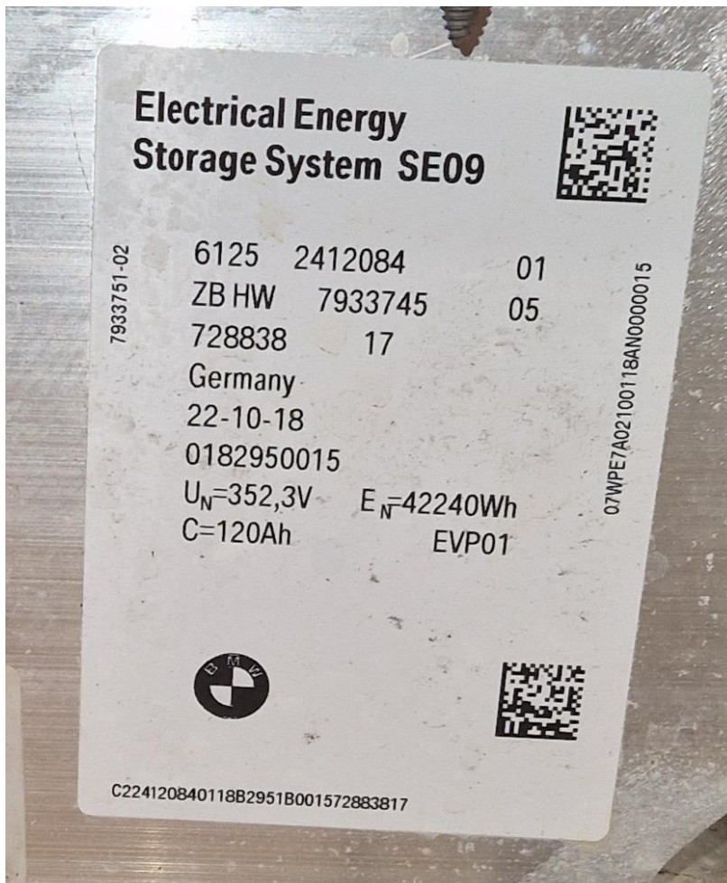
Obrázok 1 Výrobný štítok EV batérie BMW i3
